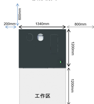
顶部视图
