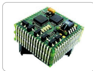
混血儿(SiP)
