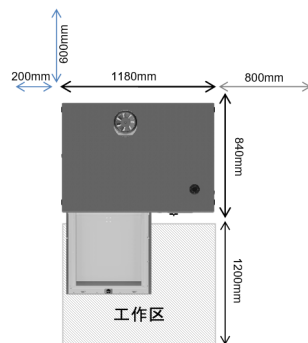
顶部视图
